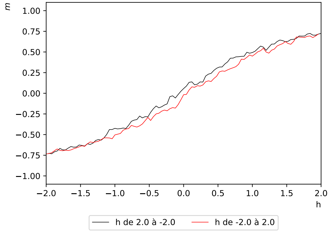
Hystérésis de l'aimantation - réseau de taille L=64 - champ magnétique d'amplitude h=2 à T=5.0
